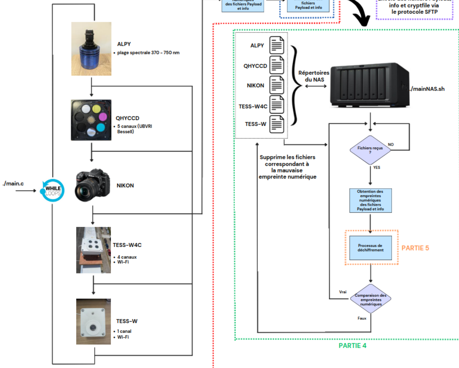
FIGURE 5 – Vue d'ensemble du fonctionnement du code d'interopérabilité
